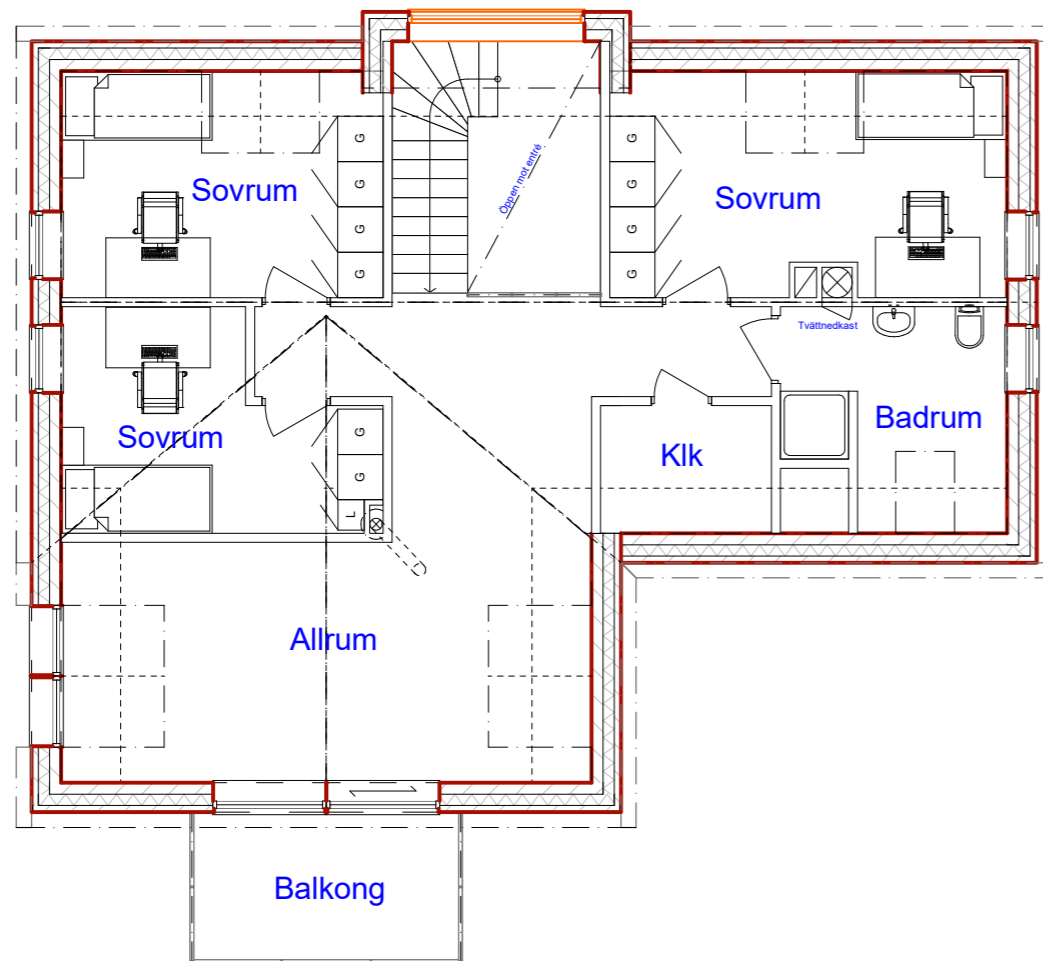
1. Vindsplan 1:100
